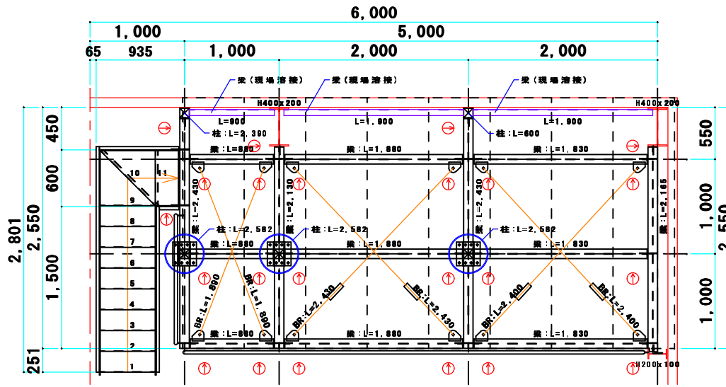
平面図 S=1/20
