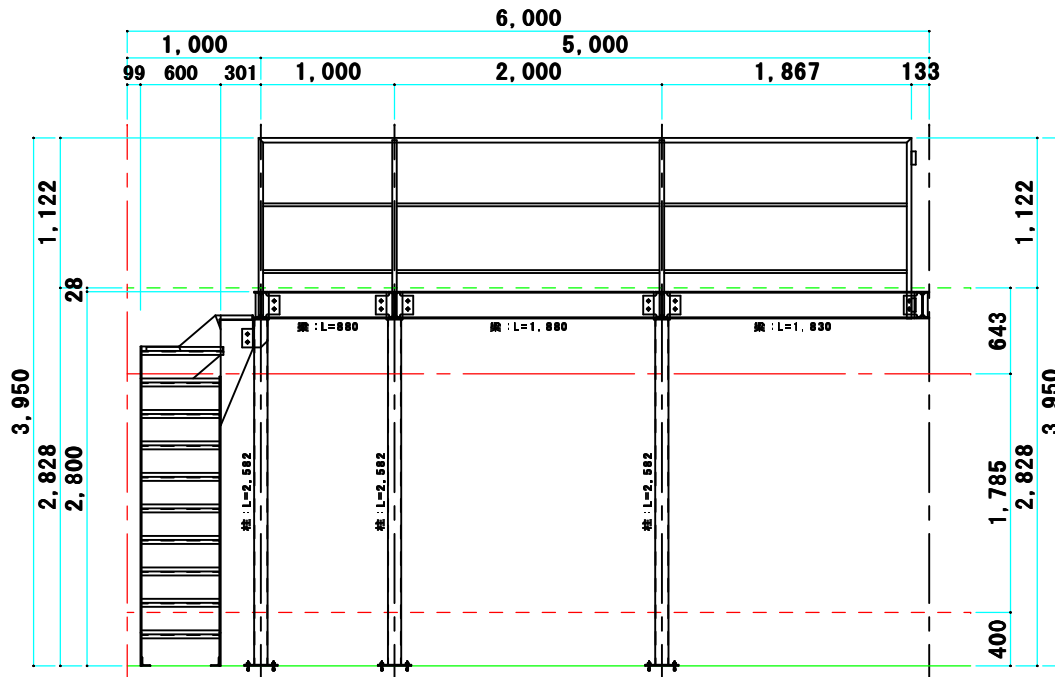
立面図 S=1/20
