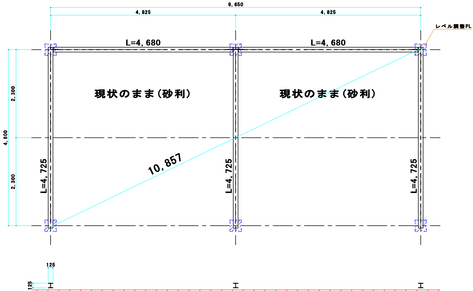
土台伏図 S=1/20
