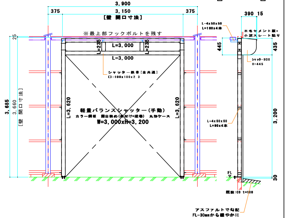
計画 立面図 S=1/20
