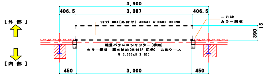
計画 平面図 S=1/20
