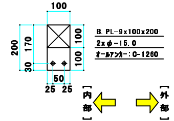
計画 平面図 S=1/20
