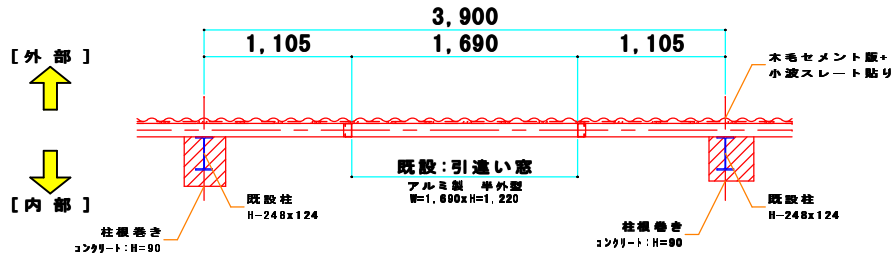
現況 平面図 S=1/20
