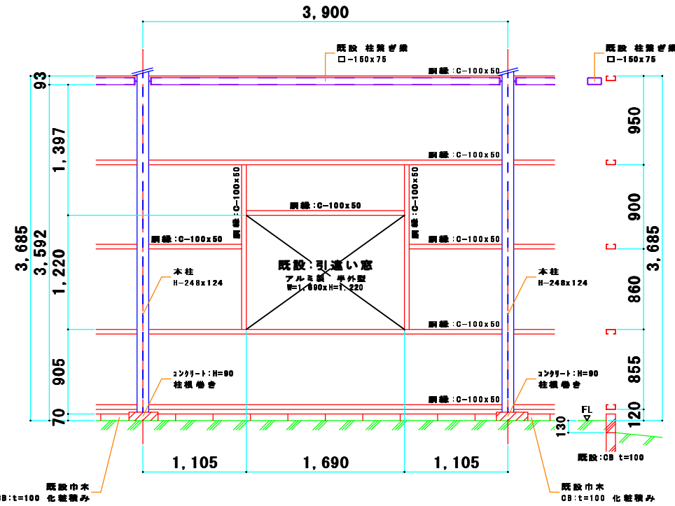
現況 立面図 S=1/20
