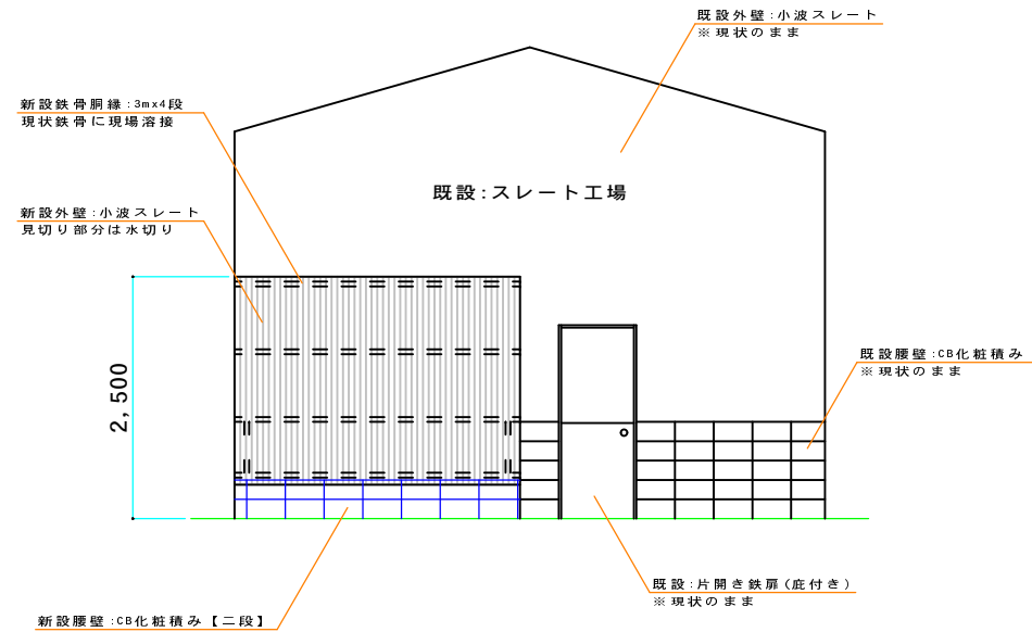
立面図 S=1/20
