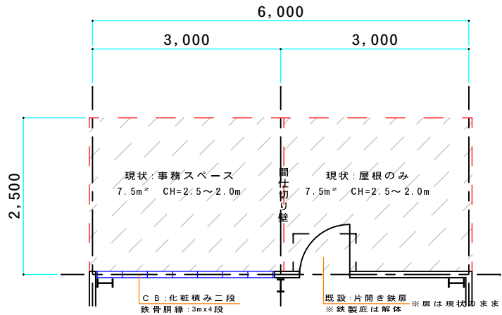
平面図 S=1/20
