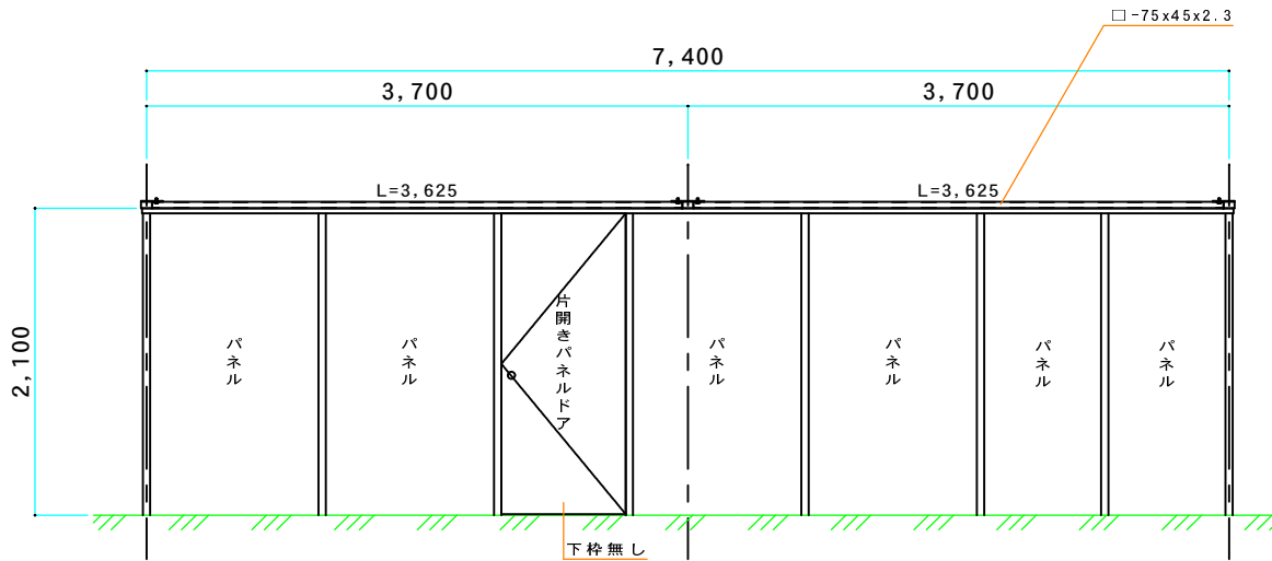
立面図 S=1/20 ※壁は全てパネル、天井は無し(オープン)
