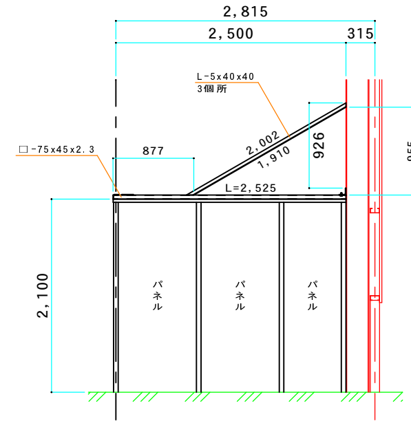
立面図 S=1/20 ※壁は全てパネル、天井は無し(オープン)
