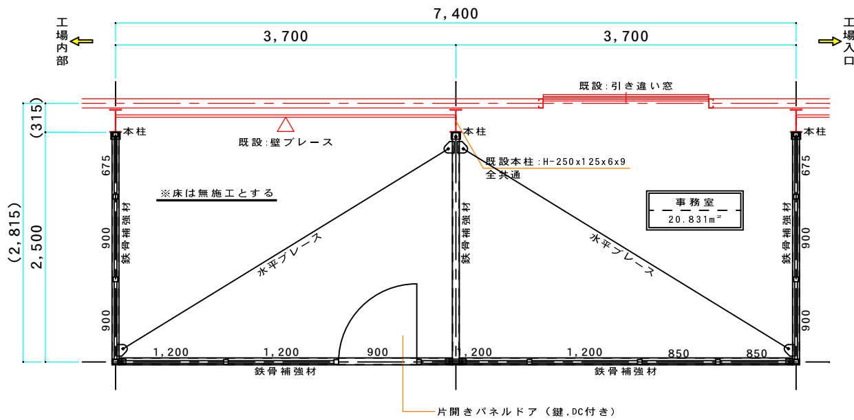
平面図 S=1/20 ※壁は全てパネル、天井は無し(オープン) 注)ポスト(パネル割)は施主様との打合せによる
